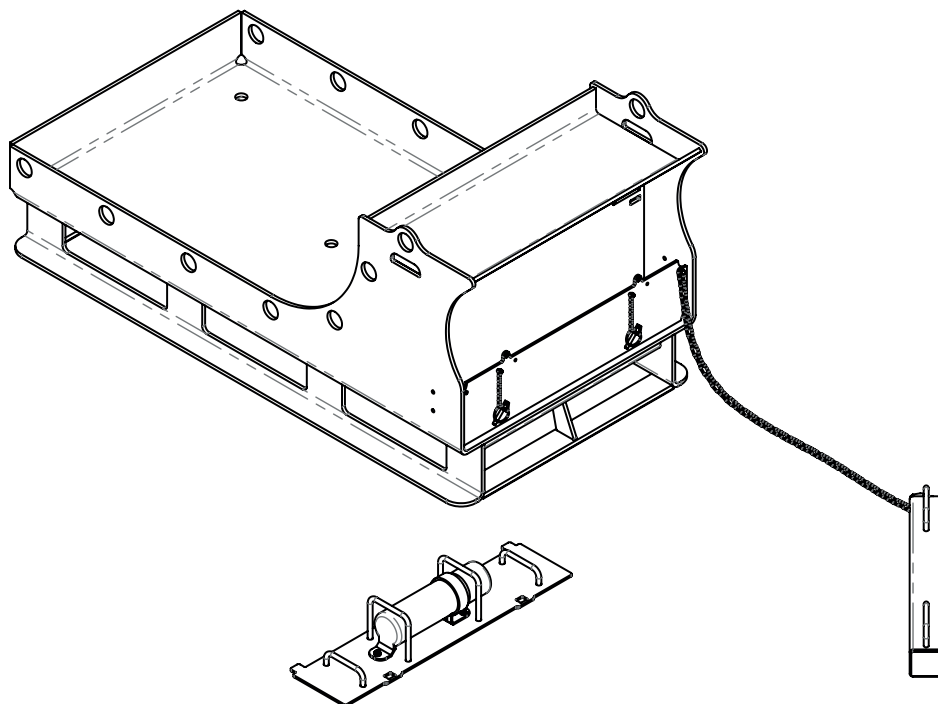
Transportgestell
