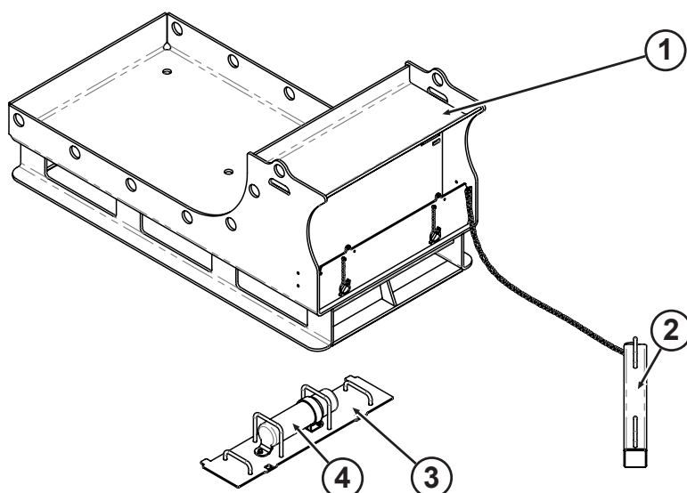
Ansicht Transportgestell
