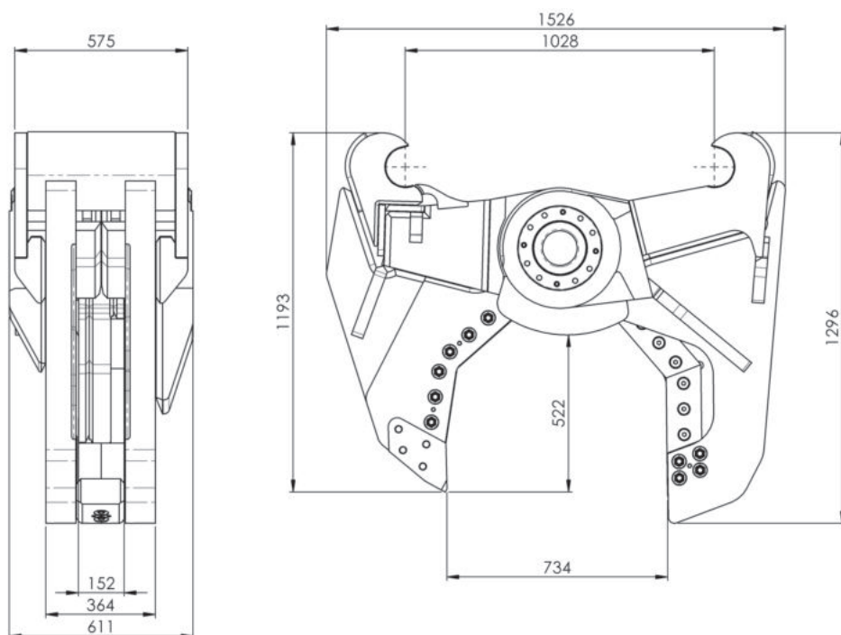
Stahl-Gebiss mit Doppelschneide
