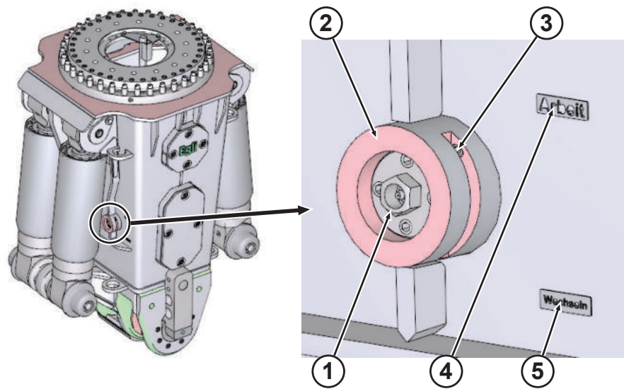
Umschaltventil für Gebisswechsel
