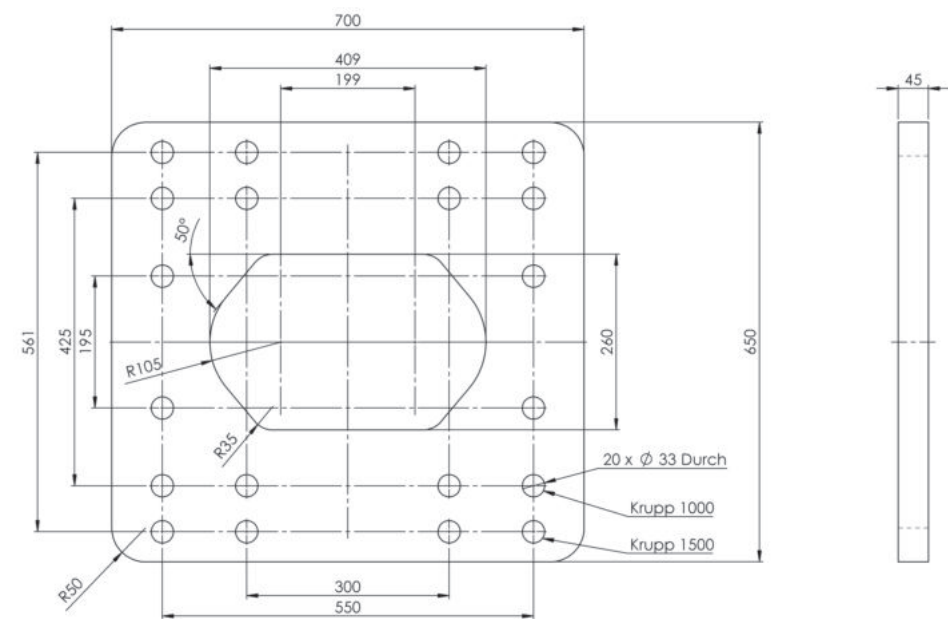
Lochbild
