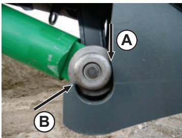
Korrekte Montage A: anliegend B: frei
