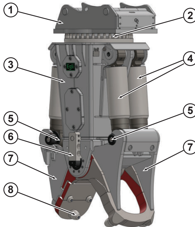
Gesamtansicht mit Gebiss
