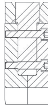
Verschraubung Spitzenmesser
