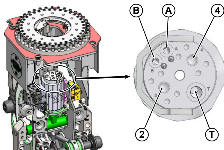
Drehdurchführung mit Anschlüssen
