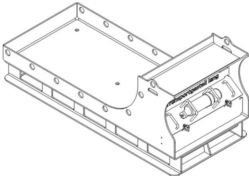
Transportgestell lang (für MultiCut-Gebiss)
