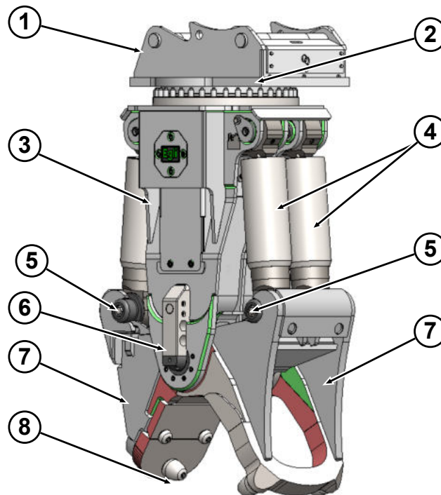
Gesamtansicht mit Gebiss
