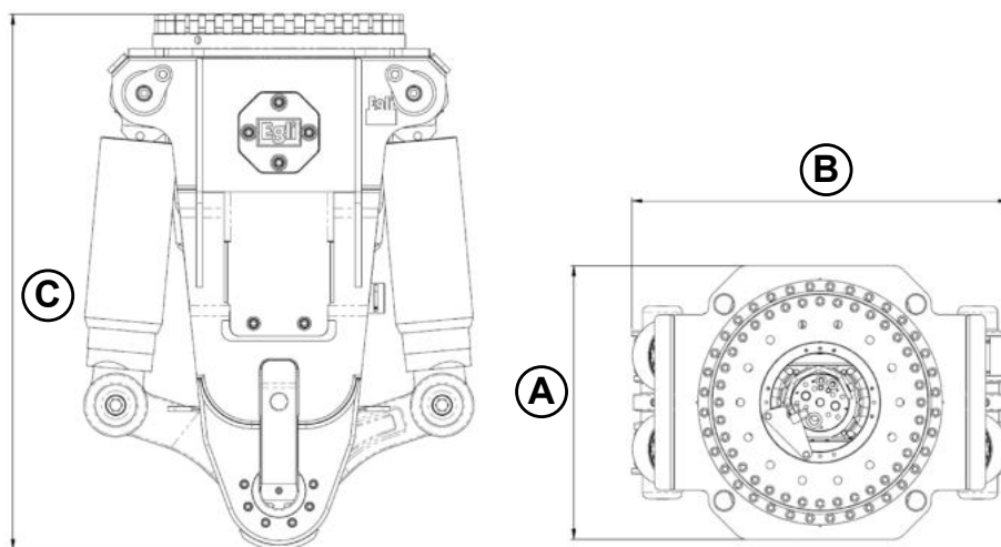
Darstellung Anbaugerät (ohne Gebiss)
