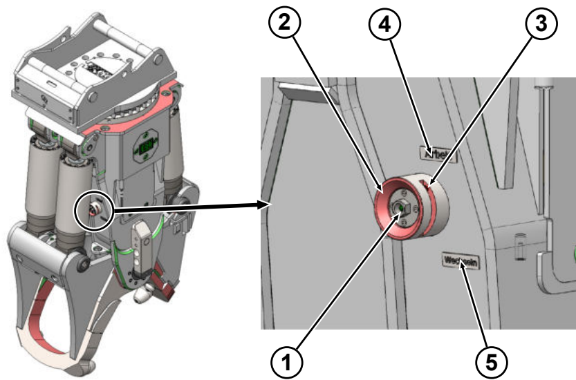
Umschaltventil für Gebisswechsel
