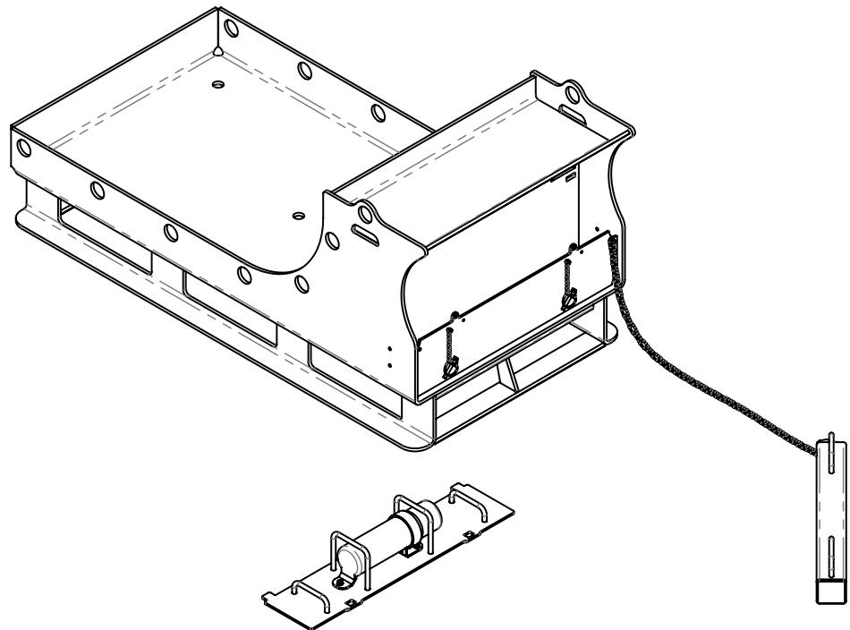
Transportgestell
