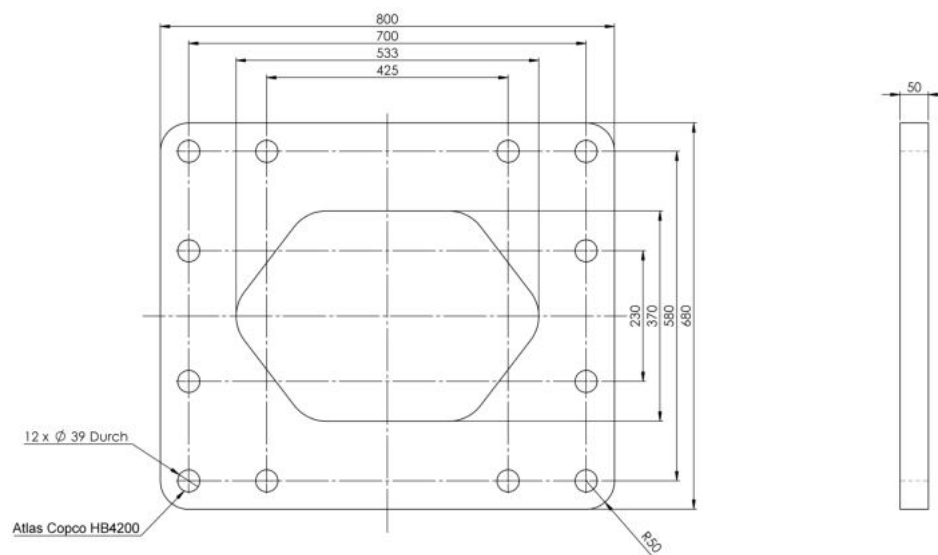
Lochbild
