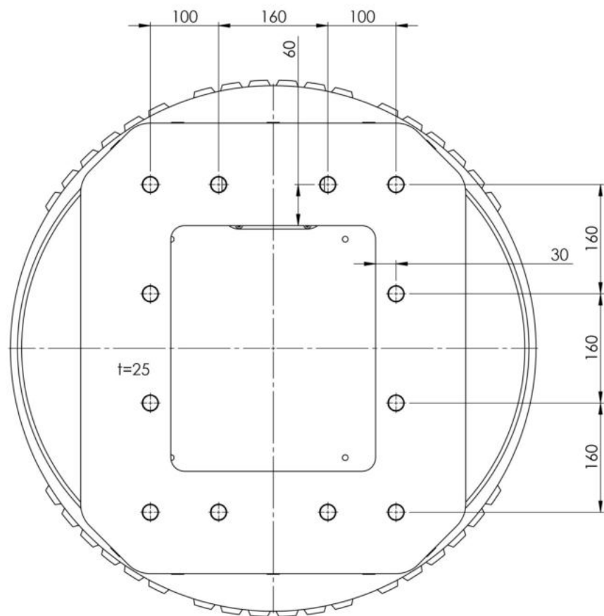
Lochbild auf der Anschraubfläche des Hydraulikmagneten
