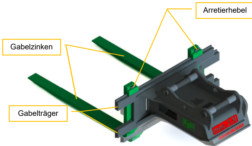
Abb. 7.3-1: Gabelzinken einstellen
