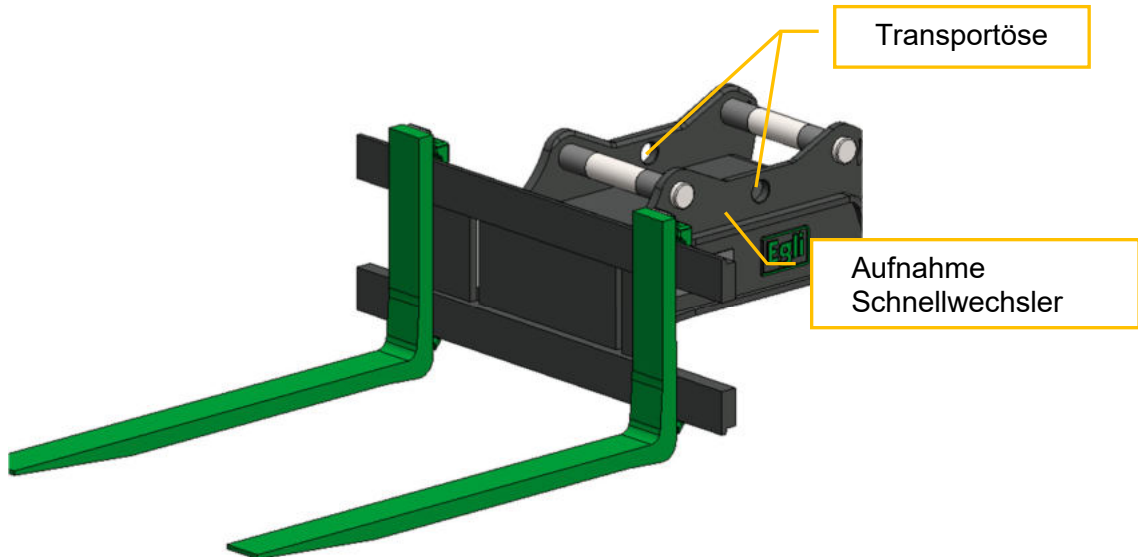
Abb. 5.1-1: Transportöse
