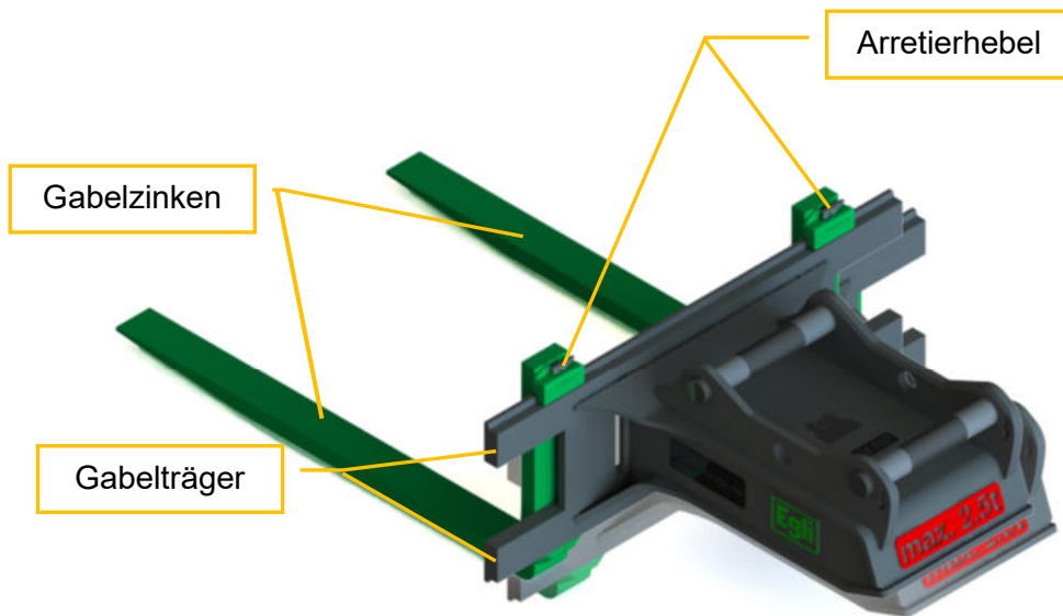
Abb. 7.3-1: Gabelzinken einstellen
